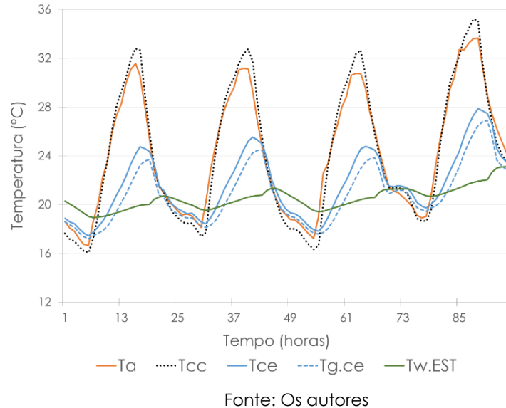
Figura 4 – Temperaturas medidas em CE, CC, EST e no ambiente externo entre 28 e 31/12/2019
